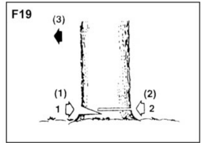
(1) Urez (2) Rez za obaranje (3) Smer obaranja stabla
